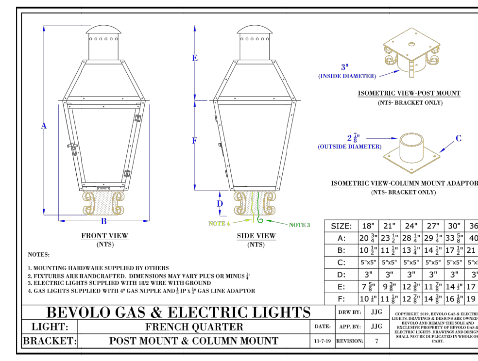
BEVOLO PIER LIGHTS
